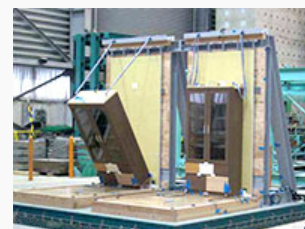
振動台実験の様子 協力：東急建設（株）技術研究所
